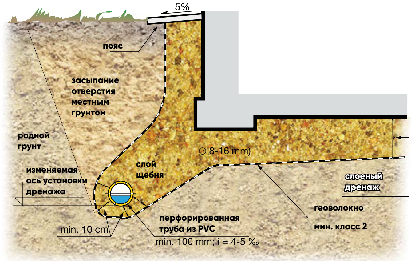
Многослойный дренаж дома из щебня и геоволокна в слабопроницаемых грунтах
