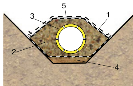
призмный дренаж
