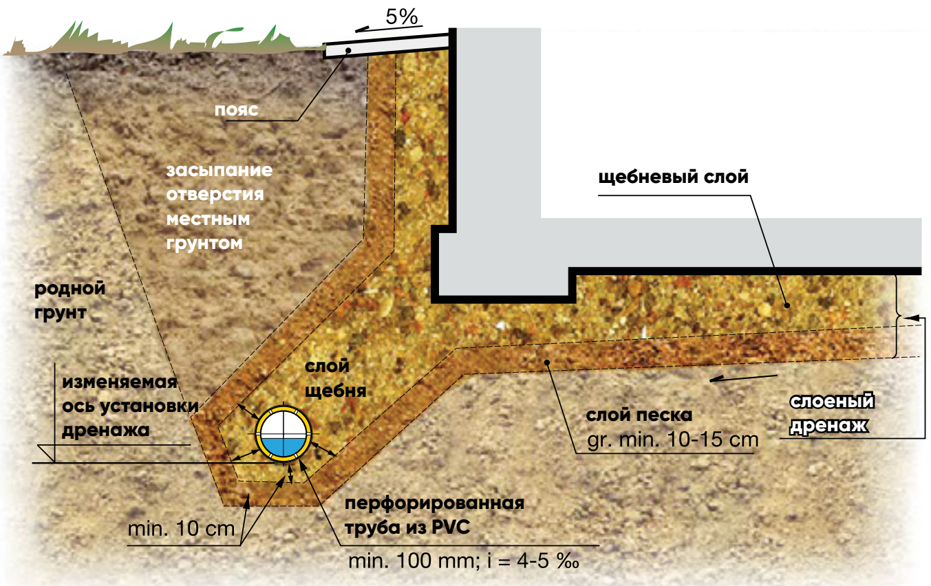
Многослойный песчано-щебневый дренаж дома в слабо проницаемых грунтах
