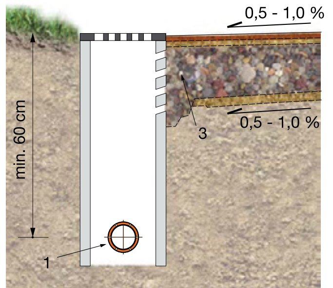
Сборный колодец, окруженный беговой дорожкой
