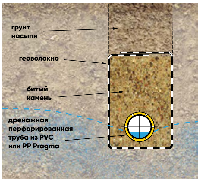
С использованием геоволокна
